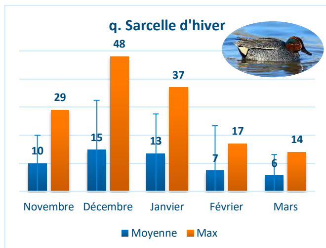
Annexe 2.3. Abondance moyenne et maximale mensuelle de 2012 à 2020 des 17 espèces d'oiseaux d'eau sélectionnées sur le site de Cadarache.
